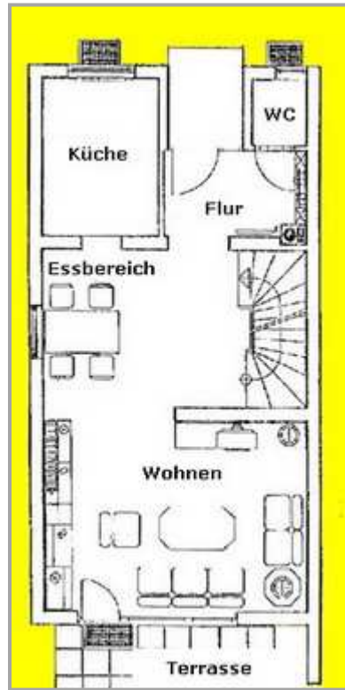
Erdgeschoss
