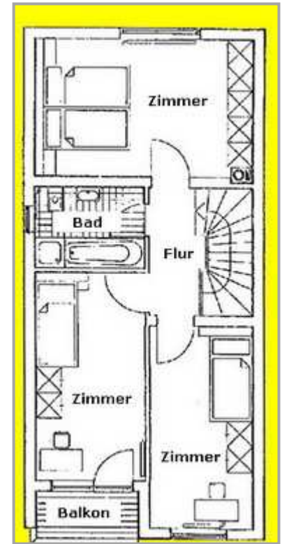
1.Obergeschoss
